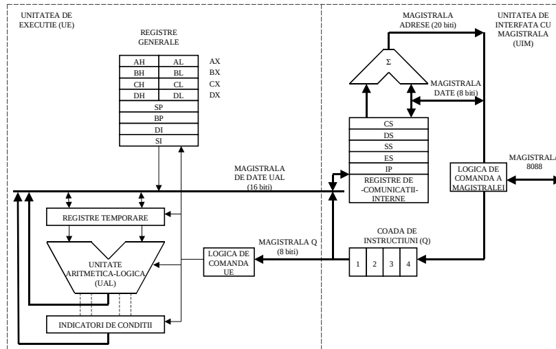
1: Schema bloc a microprocesorului 8088
