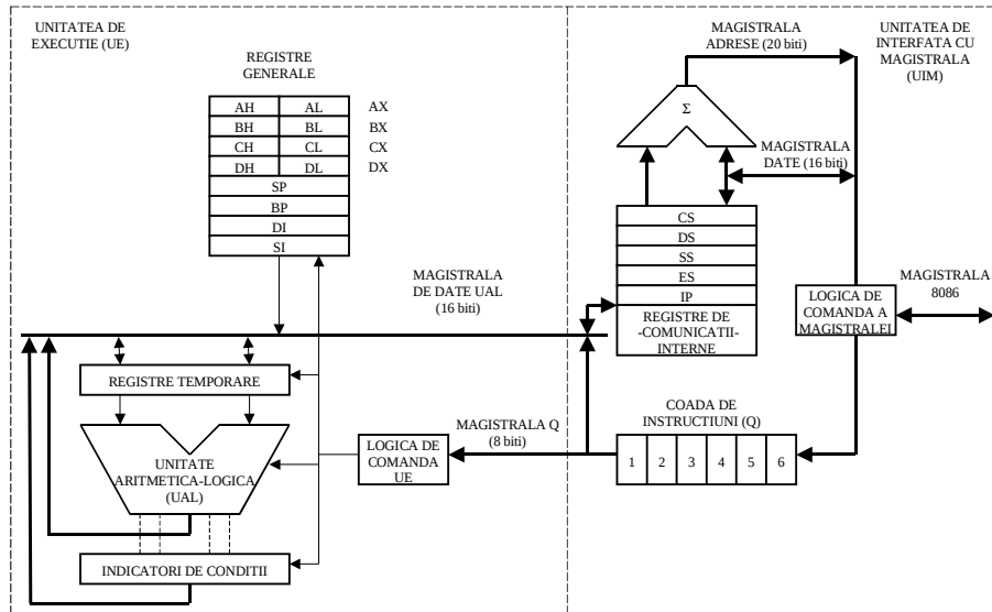
Figura 1: Schema bloc a microprocesorului 8086
